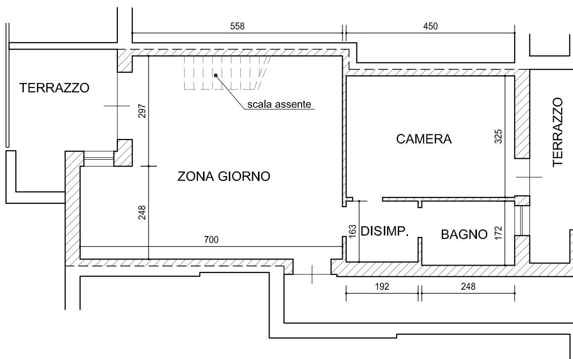
PIANO SECONDO h= 2.70
