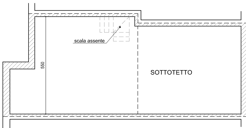
PIANO TERZO h max (colmo) = 2.40
